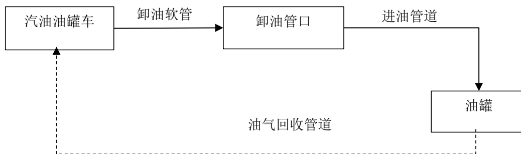
图 2-1 汽油卸油工艺框图
