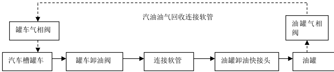
图 2-2 汽油卸油工艺流程示意图
