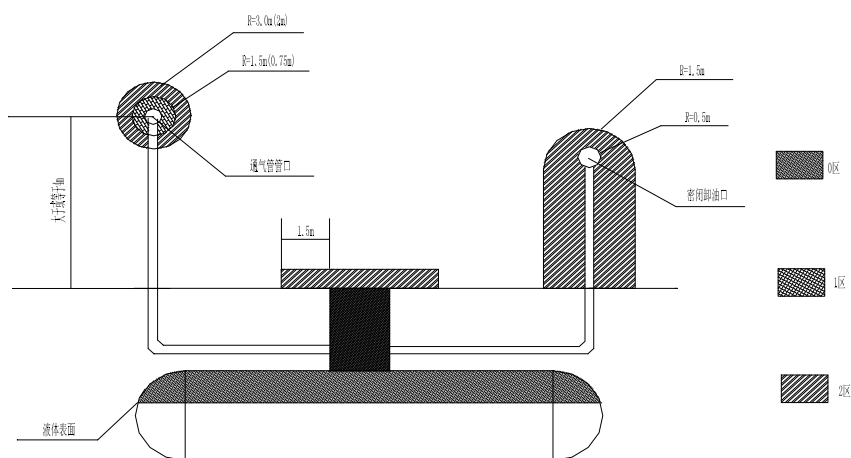
图 3-2 油罐车卸油爆炸危险区域划分
