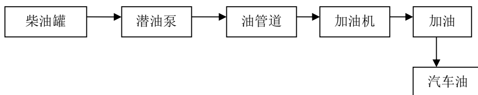
图 2-3 柴油加油工艺流程框图
