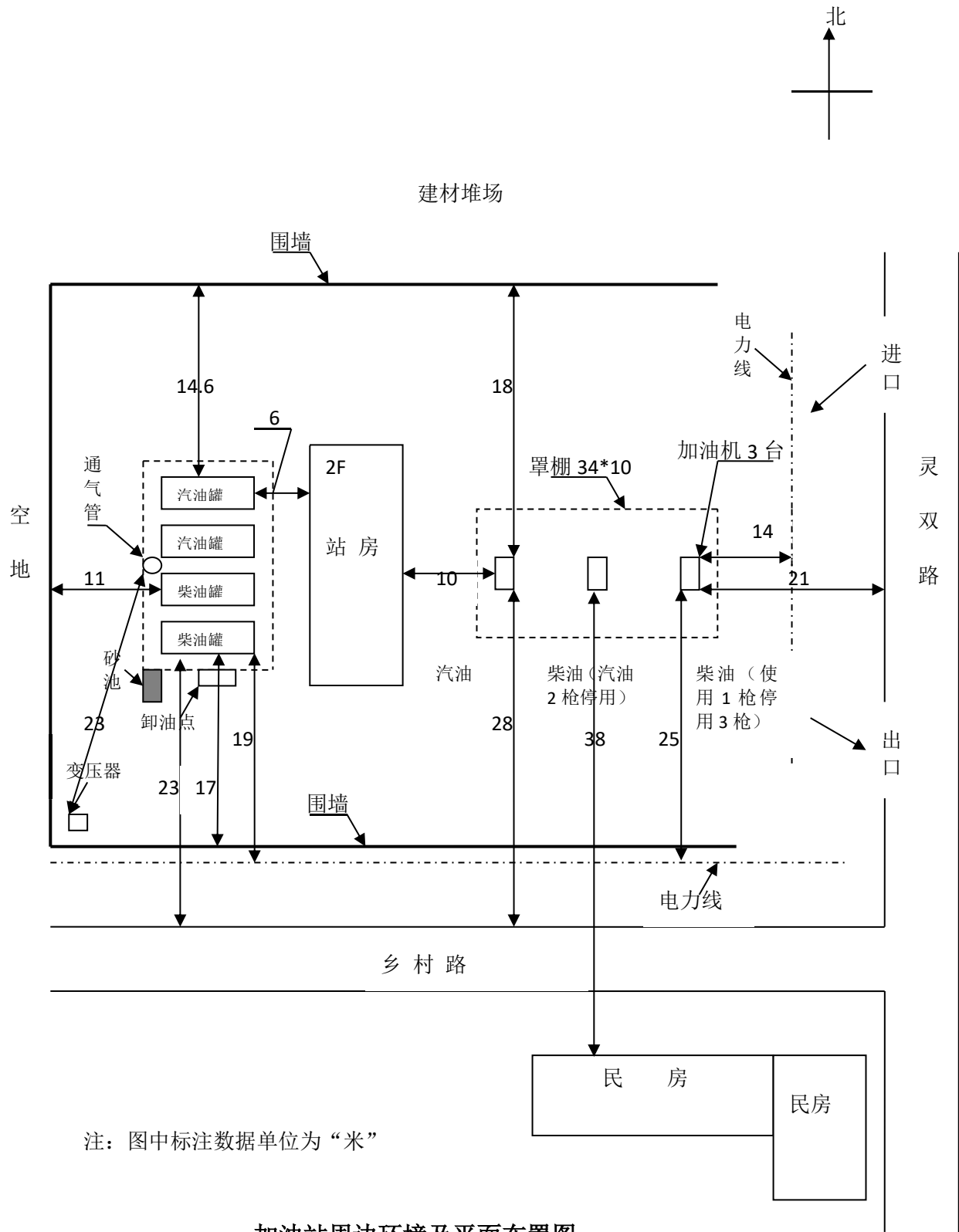
加油站周边环境及平面布置图
