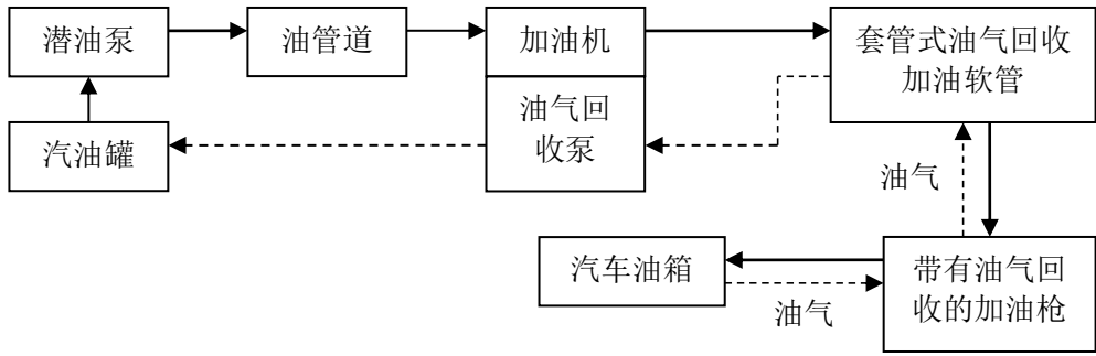
图 2-4 汽油加油及加油油气回收工艺流程框图
