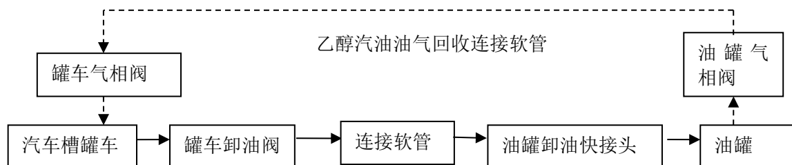
图 2-1 汽油卸油工艺流程框图
