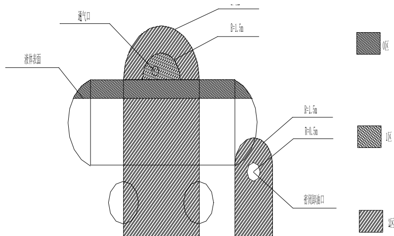
图 3-2 油罐车卸油爆炸危险区域划分
