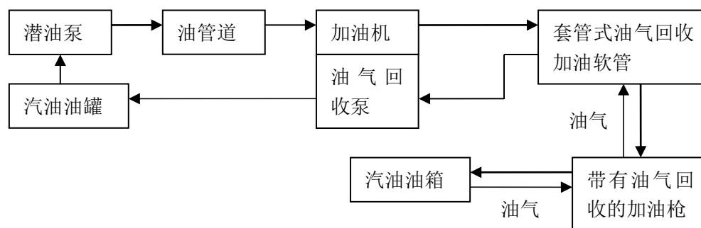
图 2-2 汽油加油及加油油气回收工艺流程示意图
