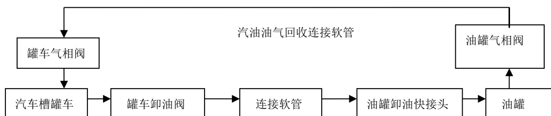
图 2-1 汽油卸油工艺流程示意图
