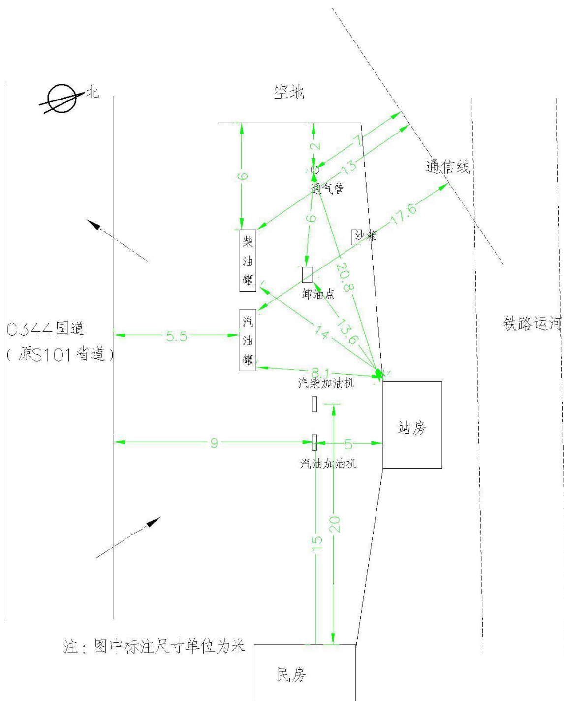
加油站周边环境及平面布置图
