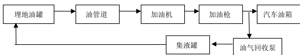
图 2-3 加油工艺流程示意图
