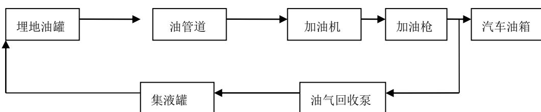
图 2-3 加油工艺流程示意图
