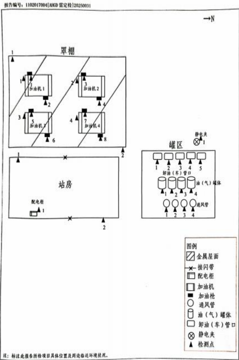
定期检测项目平面布置图
