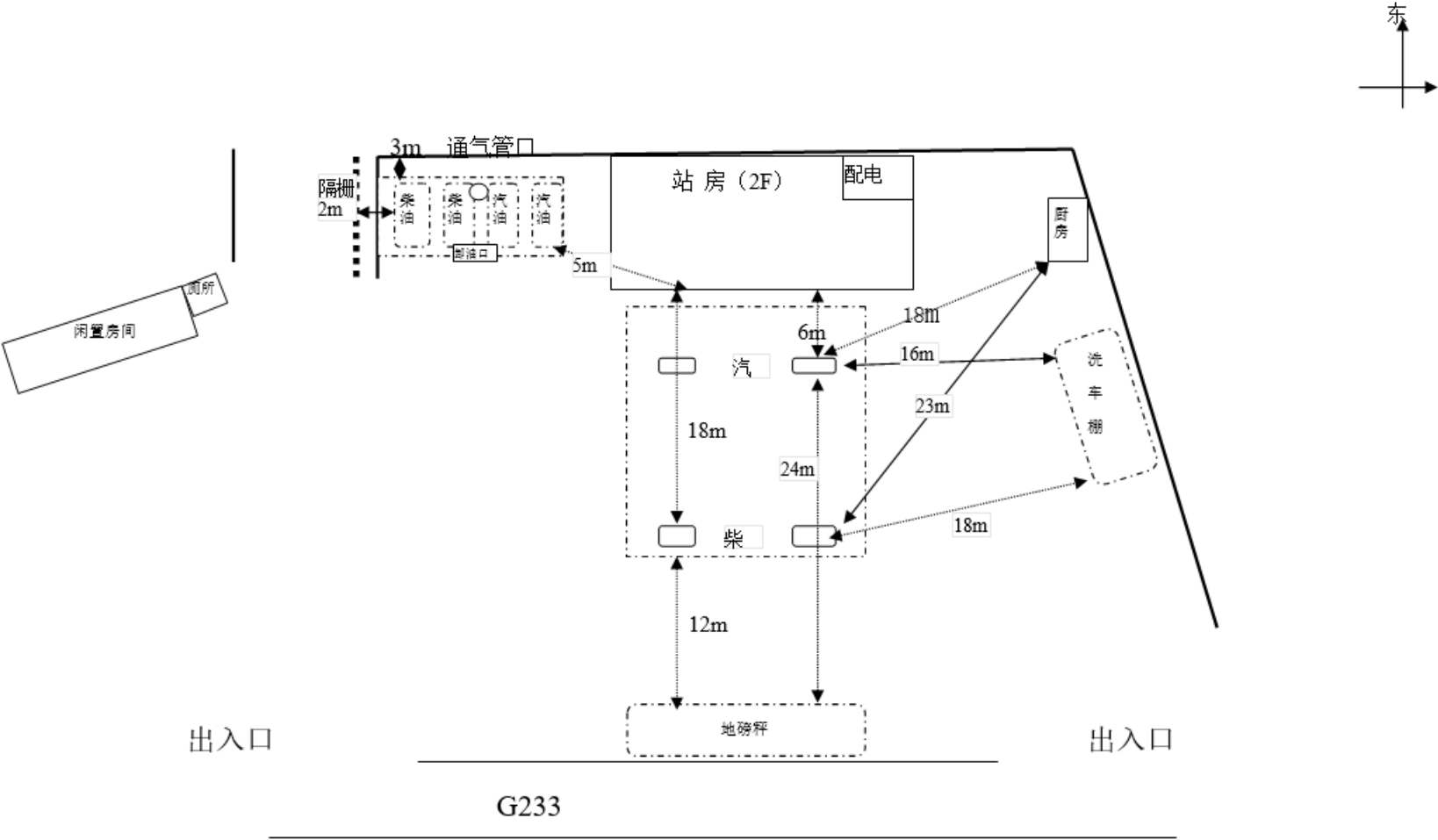
9.1 总平面布置示意图（2025.04）
