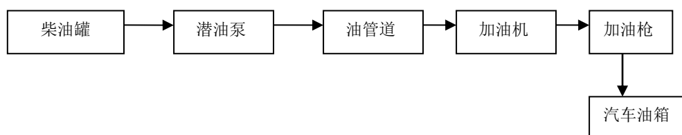
图 2-3 柴油加油工艺流程图
