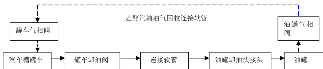
图 2-2 乙醇汽油卸油工艺流程示意图
